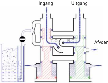
Schema bedrijfsstroom
