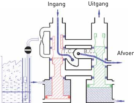
Schema snelle spoeling
