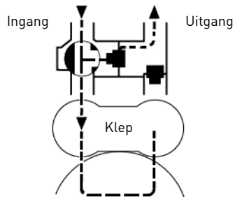
Regeneratie. Klep automatisch open voor bypass van onbehandeld water
