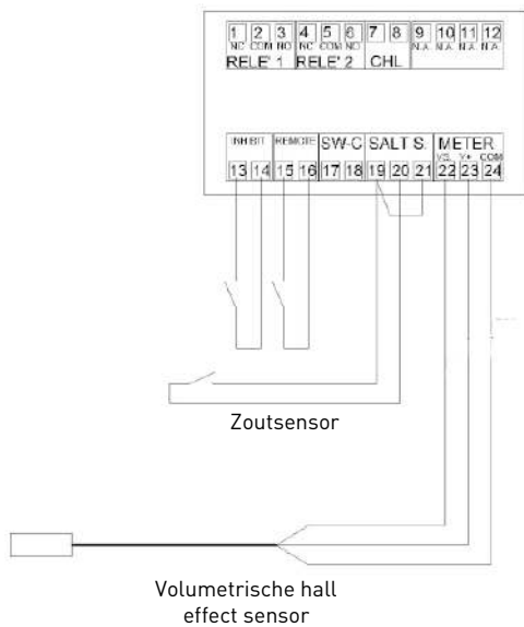
Printplaat
