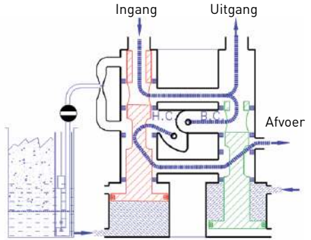
Schema terugspoelingsstroom
