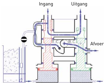
Schema trage spoeling
