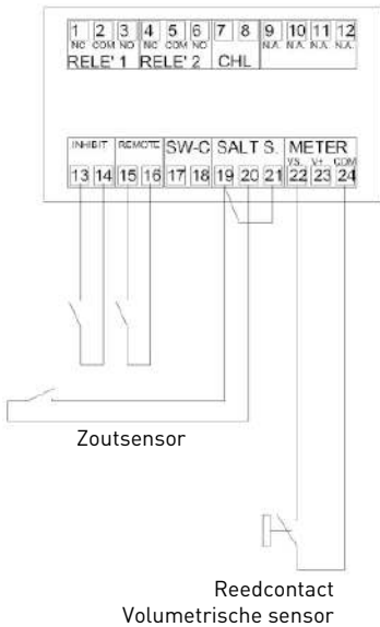
Printplaat
